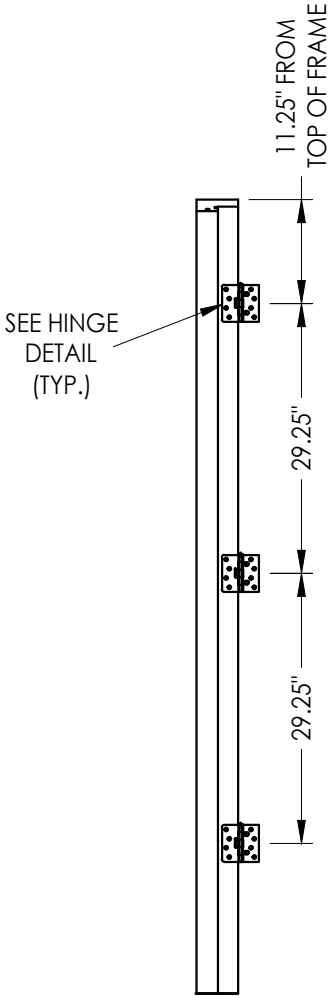
HINGE JAMB
